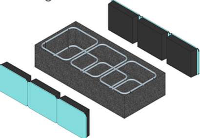
3. Add geotextile
